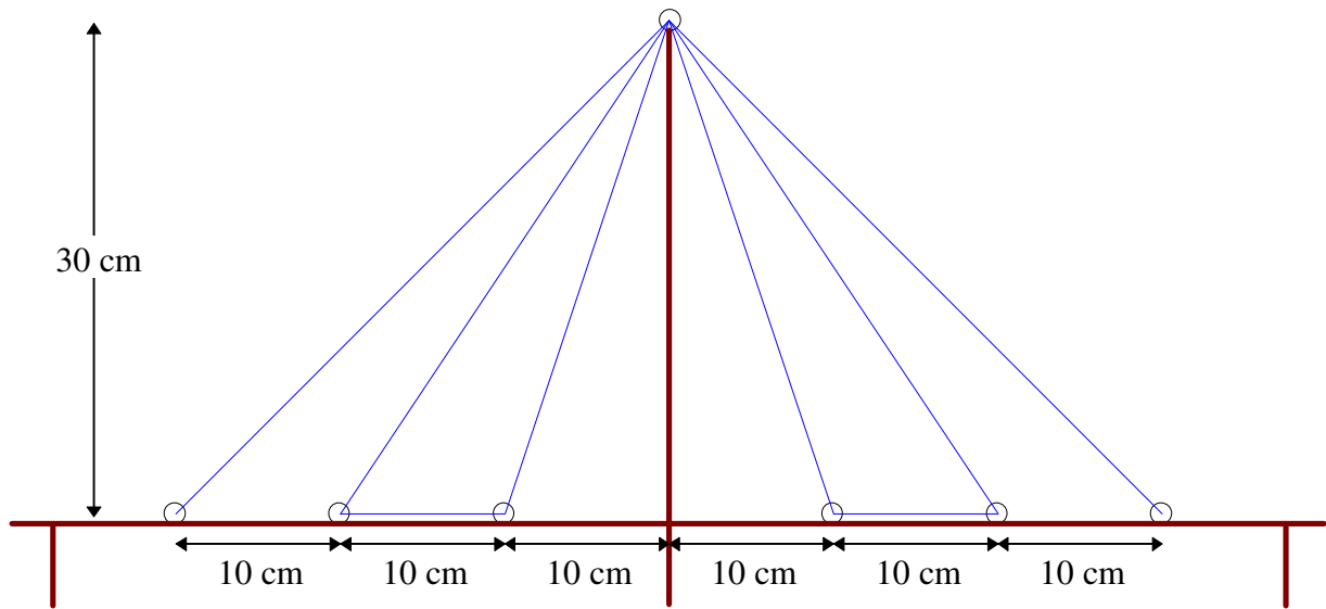
Skizze der Brücke im Maßstab 1:5
